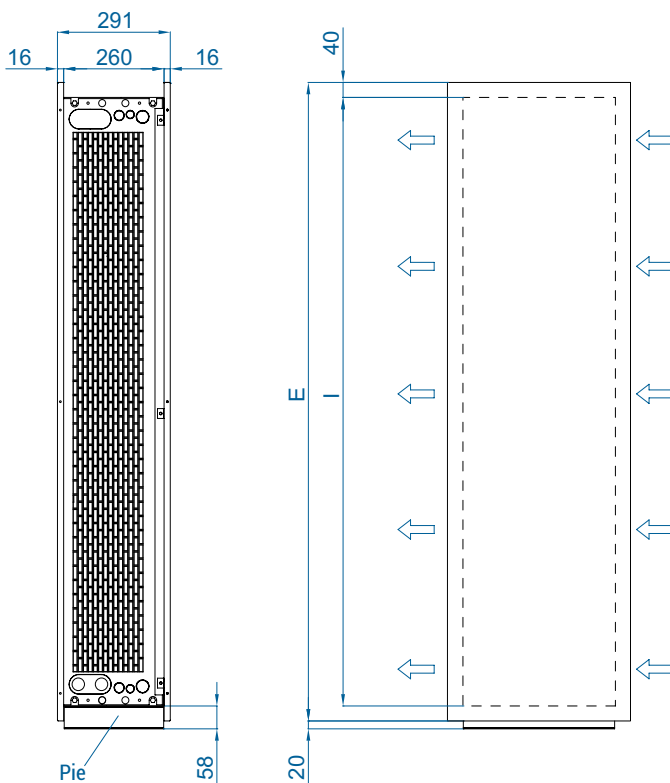
Instalación vertical
