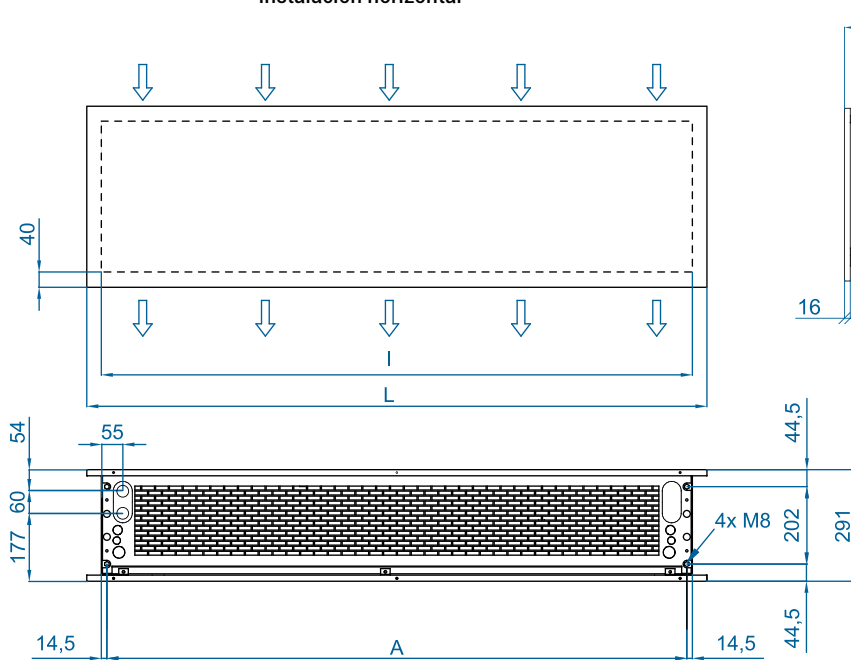
Instalación horizontal
